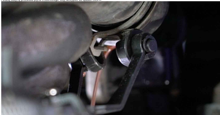
8 Odłącz przewód płynu chłodniczego.
